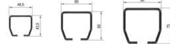
TIPO 1 PUERTAS HASTA 348kg TIPO 2 PUERTAS DE 350kg HASTA 679kg TIPO 3 PUERTAS DE 680kg HASTA 1200kg
