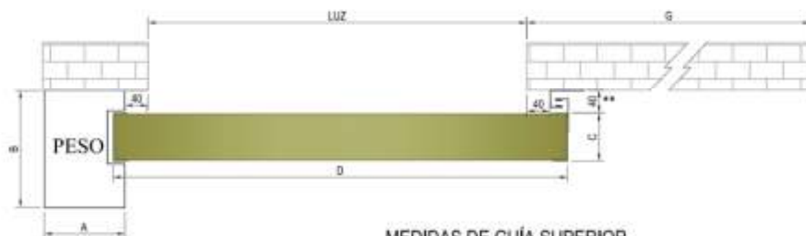
MEDIDAS DE GUÍA SUPERIOR (EN FUNCIÓN DEL PESO DE LA HOJA)
